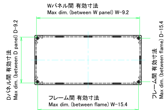
下カバー / Bottom cover
